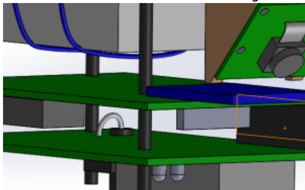
Detailansicht: Koaxkabeldurchführung
